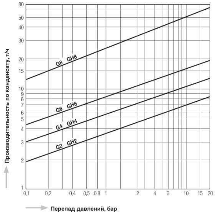
График производительности
